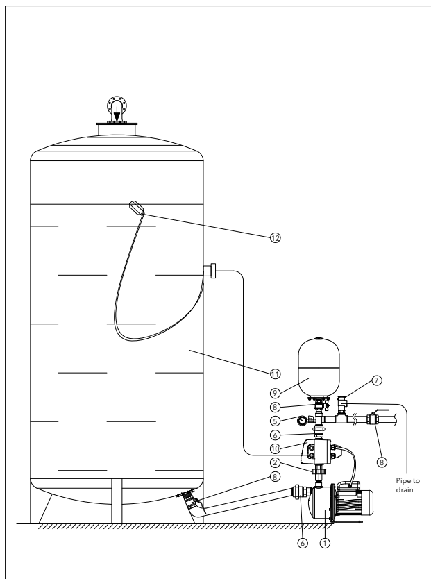
Figura 2: Configuración del sistema de agua de represurización
