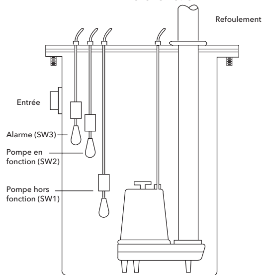
Système à pompe simple ①
